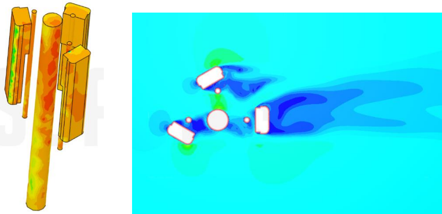
Simulation der Windlast für eine typische Mastbelegung mit CFD (Computational Fluid Dynamics)
