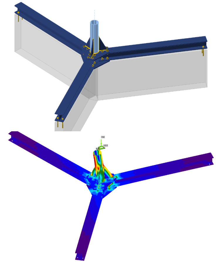
Analyse Standard Tripodmast mit CBFEM Programm Idea Statica
