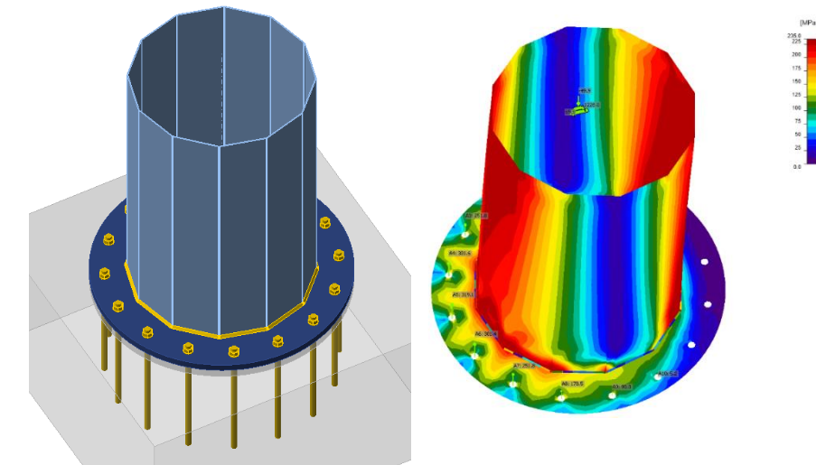
Analyse Fussverankerung Polygonrohr
