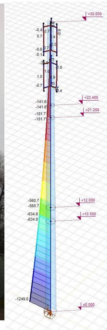
30m Monopole mit Polygonrohr
